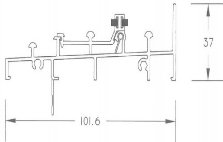
QUANTUM SLIDING DOOR SILL
